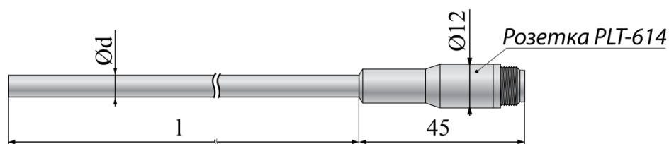
Рисунок А.3 - ПТСВ-1, ПТСВ-3, ПТСВ-4, ПТСВ-5, ПТСВ-9, ПТСВ-10, ПТСВ-11, ПТСВ-12, ЭТС
