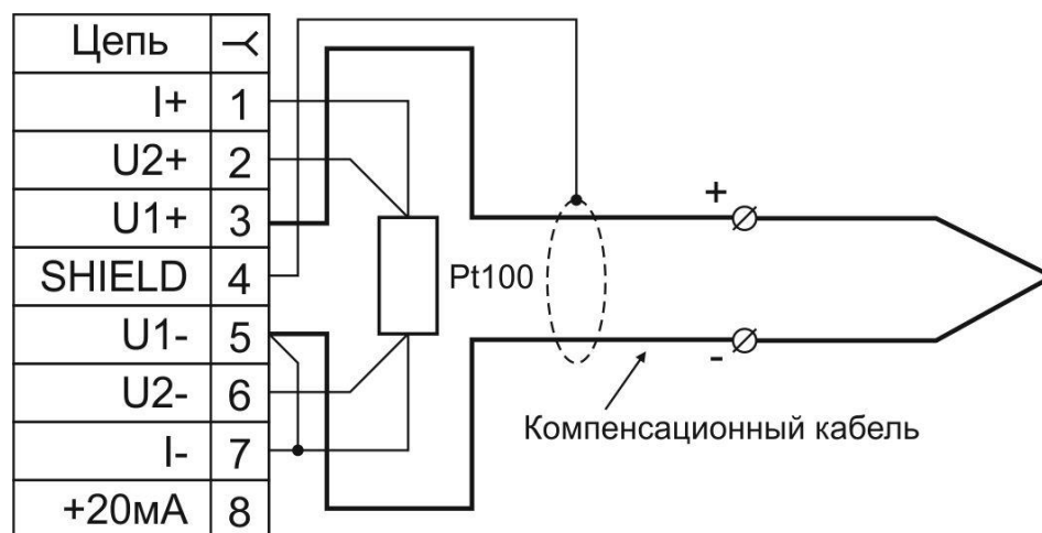
Рисунок Б.3 – Соединительный кабель № 03 для подключения термопреобразователей термоэлектрических ХА(К) и ХК(Л). Компенсационный кабель с компенсатором холодного спая, установленным в разъеме.
